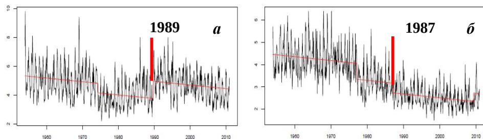
Р и с . 2 . Сдвиг в среднемесечной скорости ветра по данным МГ Черноморское (а), обусловленный переносом пункта наблюдения, и сдвиг по МГ Феодосия (б), обусловленный изменением степени защищенности метеоплощадки.
