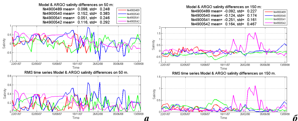
Р и с . 4. Временные ряды невязок солёности и СКО на горизонте 50 (а) и 150 м (б).
