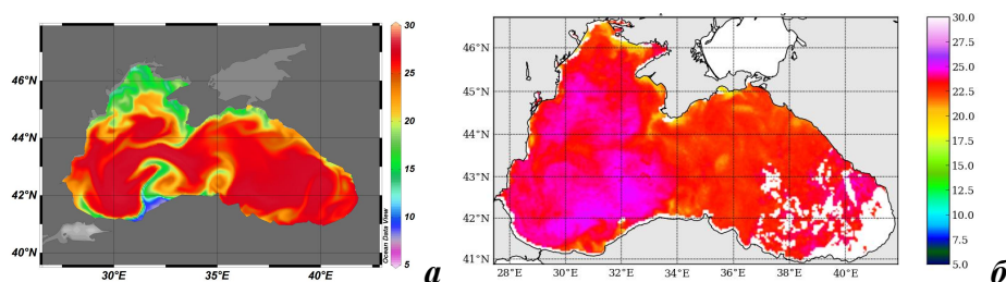
Р и с . 2 . Температура поверхности моря 8 июля 2008 г. по модельным (а) и спутниковым (б) данным.
