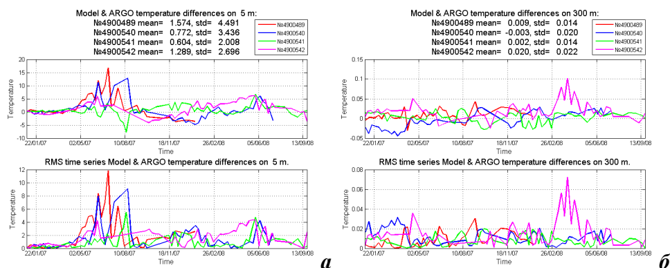
Р и с . 3. Временные ряды невязок температуры и СКО на горизонте 3 (а) и 300 м (б).
