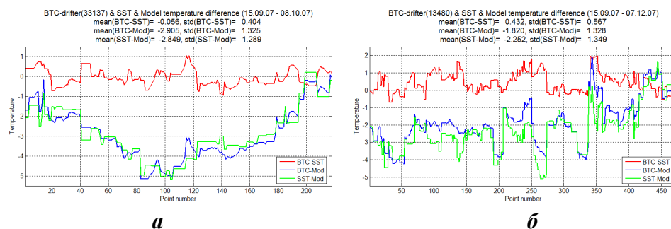
Р и с . 1 . Разница между (BTC-SST), (BTC-Mod) и (SST-Mod) на поверхности моря по данным буёв № 33137 (а) и № 13480 (б).
