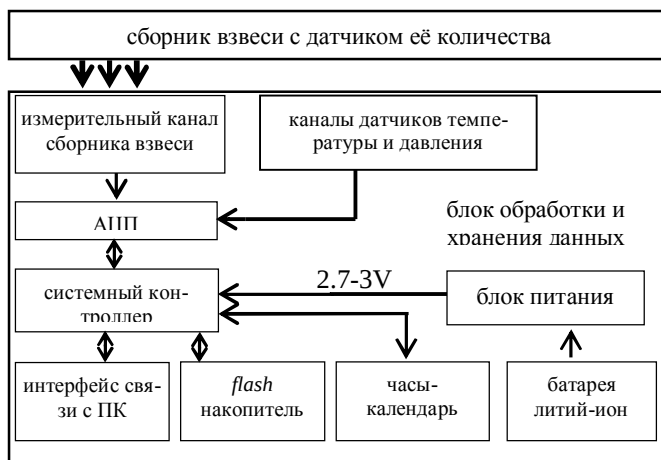
Р и с . 7. Внешний вид и структурная схема автономной ловушки взвеси.
