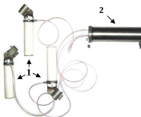
Р и с . 2 . Модуль сборников взвеси: накопительные стаканы с датчиками уровня (количества) взвеси (1); блок обработки (2).
