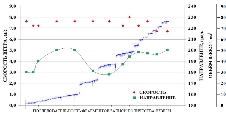
Р и с . 4 . Динамика накопления взвеси в стакане ловушки.
