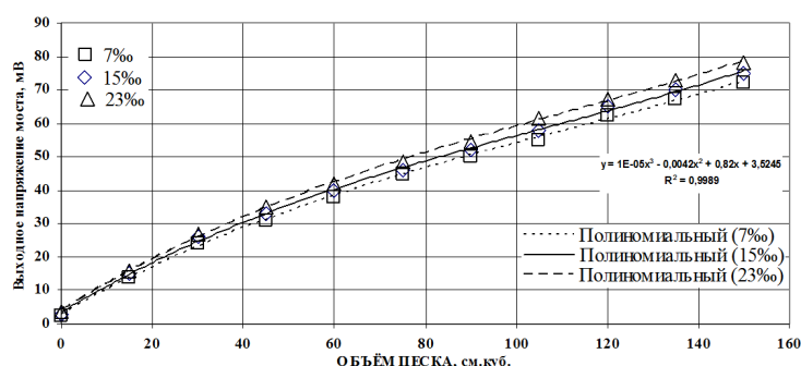
Р и с . 3 . Градуировочная характеристика ловушки.
