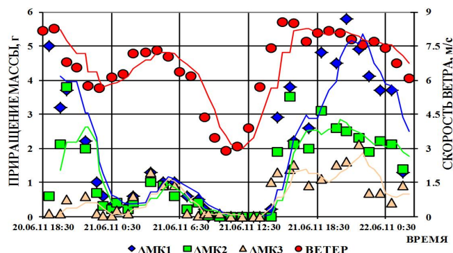
Р и с . 5. Изменение во времени скорости накопления взвеси \Delta MK1 , \Delta MK2 , \Delta MK3 в накопительных стаканах ловушек на горизонтах 0,25; 0,35 и 0,45 м у дна и скорости ветра.
