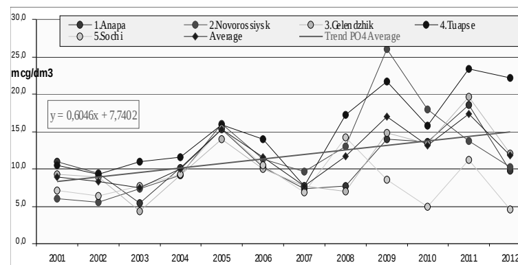
Р и с . 4. Динамика средней концентрации фосфатного фосфора P-PO_4 (мкг/дм 3 ) в прибрежных водах российской части Черного моря в 2001 – 2012 гг.
