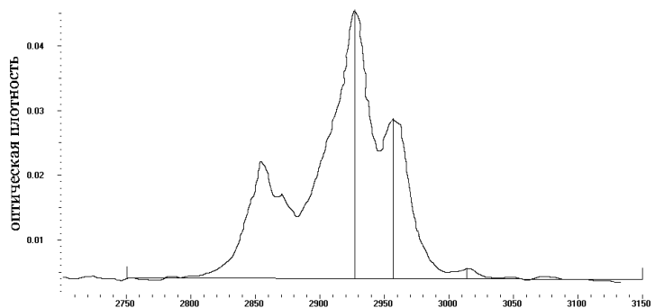
Р и с . 2 . Типичный ИК-спектр нефтяных углеводородов в период наблюдения.
