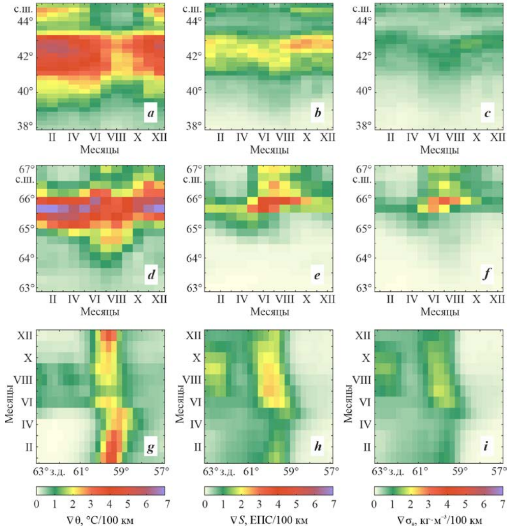
Рис. 5. Сезонная изменчивость градиентов потенциальной температуры \nabla\theta (a, d, g), солёности \nabla S (b, e, h) и аномалии потенциальной плотности \nabla\sigma_\theta (c, f, i) на меридиональных разрезах вдоль 61° з. д. в районе 1 северного участка Гольфстрима (a, b, c), вдоль 34° з. д. в районе 4 прибрежного Восточно-Гренландского течения (d, e, f) и на зональном разрезе вдоль 59° с. ш. в районе 3 фронтальной зоны Лабрадорского течения (g, h, i)
