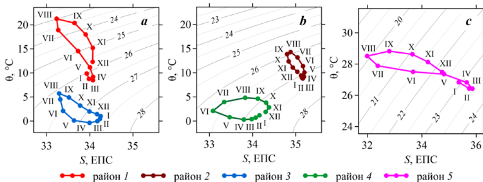
Рис. 4. TS-диаграммы сезонной изменчивости температуры и солёности на глубине 0.5 м в районах 1, 3 (а), 2, 4 (b), 5 (с)
