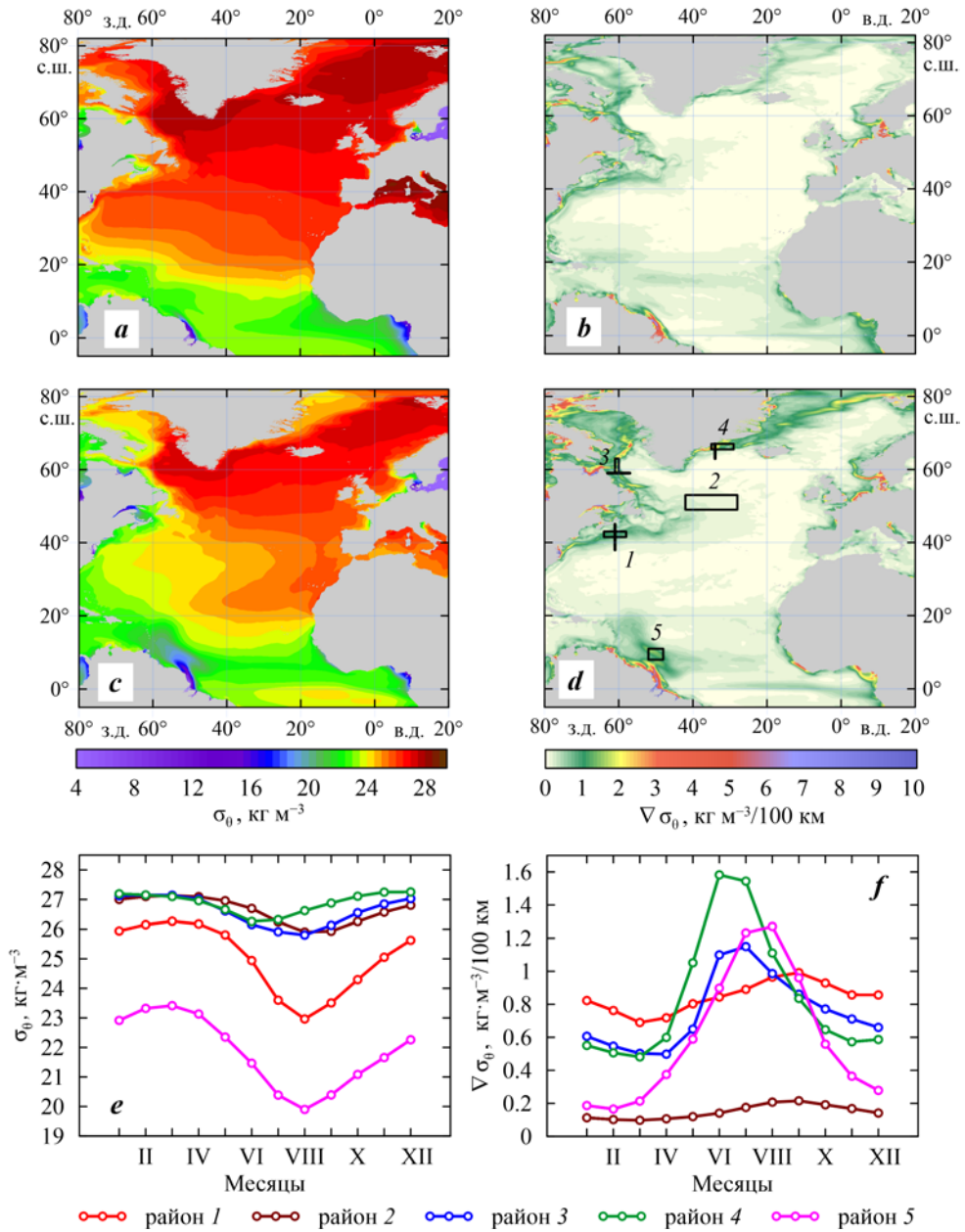
Р и с . 3 . Пространственное распределение аномалии потенциальной плотности \sigma_\theta (a, c) и горизонтальных градиентов потенциальной плотности \nabla \sigma_\theta (b, d) на глубине 0.5 м в зимний (a, b) и летний (c, d) сезоны; сезонная изменчивость средних значений \sigma_\theta (e) и \nabla \sigma_\theta (f) в районах 1–5
