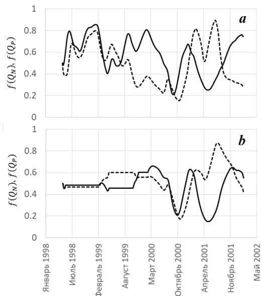
Рис. 6. Временная изменчивость функций f(Q_N) (сплошная линия) и f(Q_P) (штриховая линия), лимитирующих рост Ericaria crinita , Gongolaria barbata (а) и Phyllophora crispa (b) в районе м. Коса Северная
