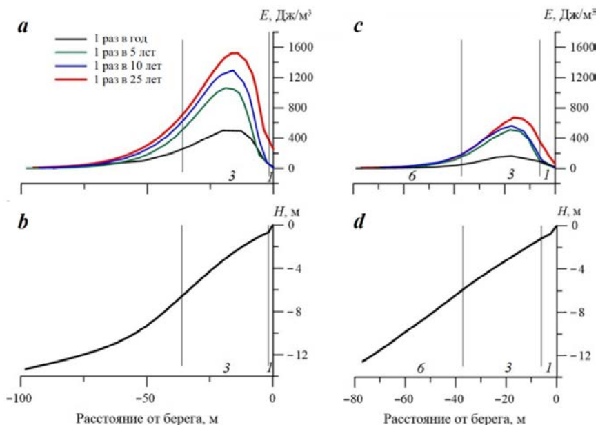
Рис. 9. Профили плотности кинетической энергии (а) и рельефа дна (б) на разрезе III; профили плотности кинетической энергии (с) и рельефа дна (д) на разрезе IV. Цифрами обозначены донные природные комплексы из работы [2]
