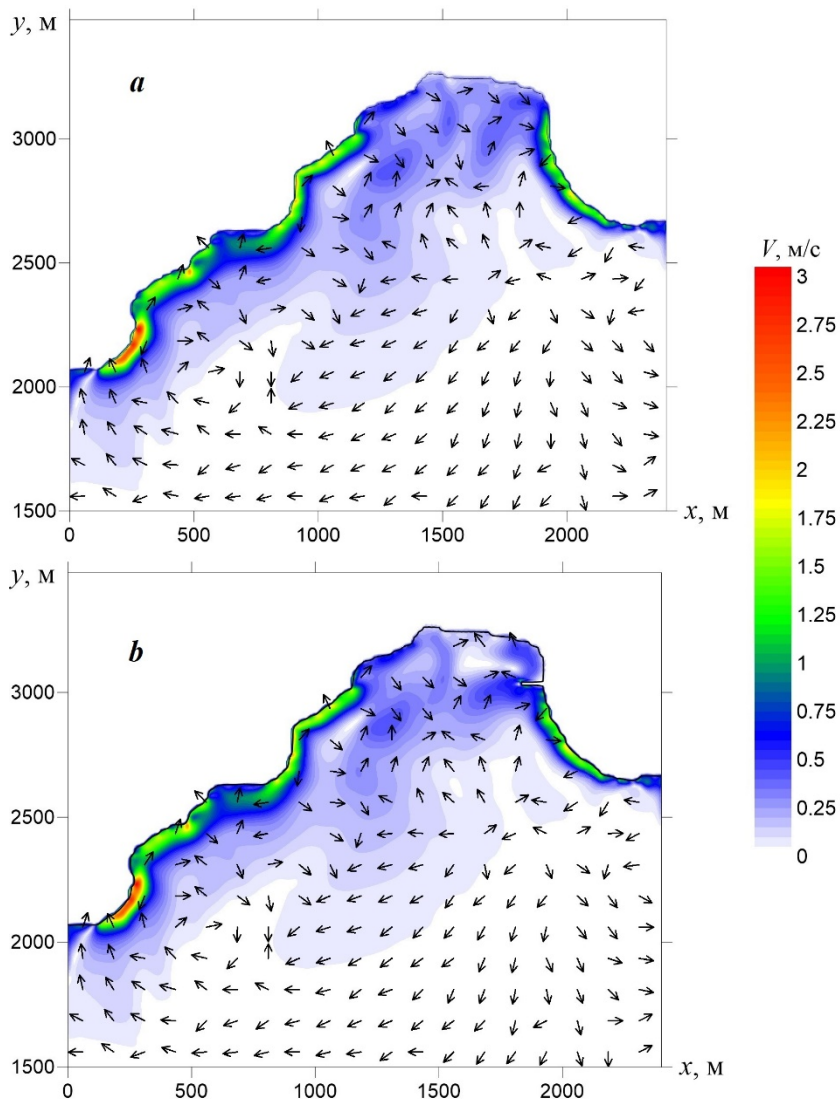
Р и с . 5 . Волновые течения в бухте Ласпи при штормах, возможных 1 раз в 25 лет, без учета гидротехнического сооружения (а), с учетом гидротехнического сооружения (b)
