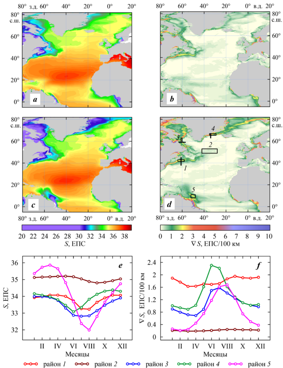
Р и с . 2 . Пространственное распределение солености S (a, c) и горизонтальных градиентов солености \nabla S (b, d) на глубине 0.5 м в зимний (a, b) и летний (c, d) сезоны; сезонная изменчивость средних значений S (e) и \nabla S (f) в районах 1–5
