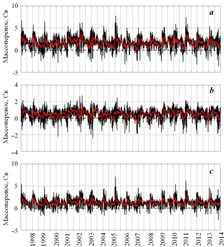
Рис. 3. Поперечный массоперенос вод (Св) в слоях: 0–200 м (а), 0–50 м (b), 50–200 м (с). Положительные значения соответствуют массопереносу в направлении от шельфа в мористую часть. Красная кривая характеризует тренд, полученный скользящей средней, с окном в 30 дней [12]
