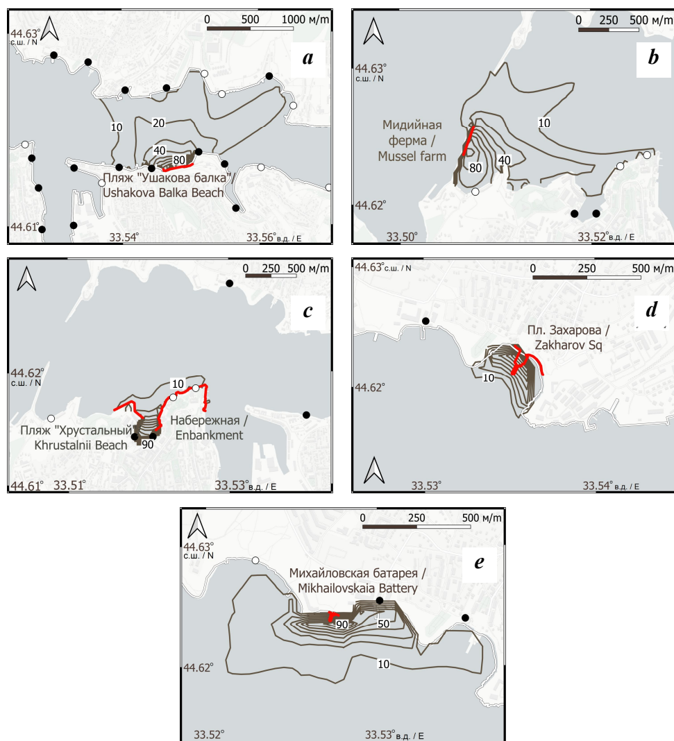
Р и с . 4 . Функция влияния для взвеси в поверхностном слое воды для пляжа «Ушакова балка» (a), мидийной фермы в Мартыновой бухте (b), центра города (c), площади Захарова (d) и Михайловской батареи (e). Изолинии проведены через каждые 10 % F i g . 4 . Influence function for suspended matter in the surface water layer for Ushakova Balka Beach (a), the mussel farm in the Martynova Bay (b), the city centre (c), Zakharova Square (d) and Mikhailovskaya Battery (e). The isolines are given for each 10 %
