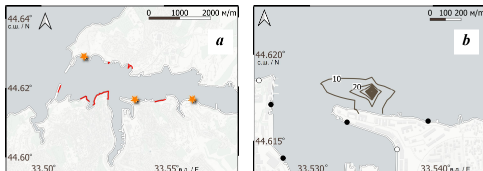
Р и с . 6 . Карта потенциально безопасного расположения дополнительных выпусков городской канализации (а) и изолинии суммарного поля концентрации консервативной примеси для точечного источника (b). Результаты модельного расчета. Изолинии проведены через каждые 10 % от максимума в точке сброса
