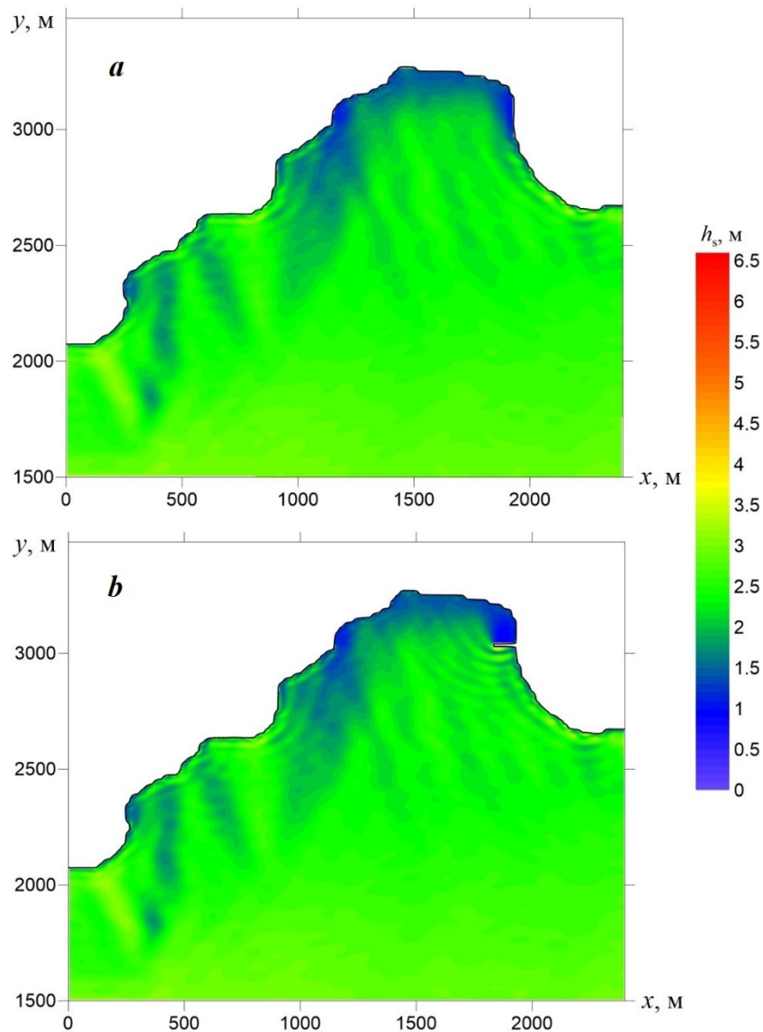
Рис. 2. Значимые высоты волн в бухте Ласпи при штормах, возможных 1 раз в год, без учета гидротехнического сооружения (а), с учетом гидротехнического сооружения (б)
